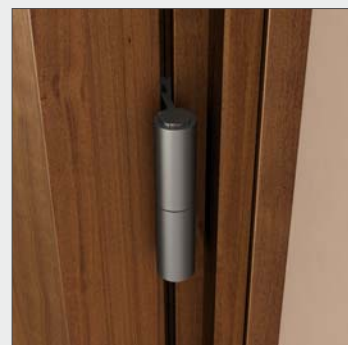
Robust hinge supporting 100kg frame. Charnière robuste de support de châssis jusqu'à 100kg.
